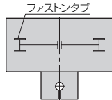
コンデンサ内部配線図
